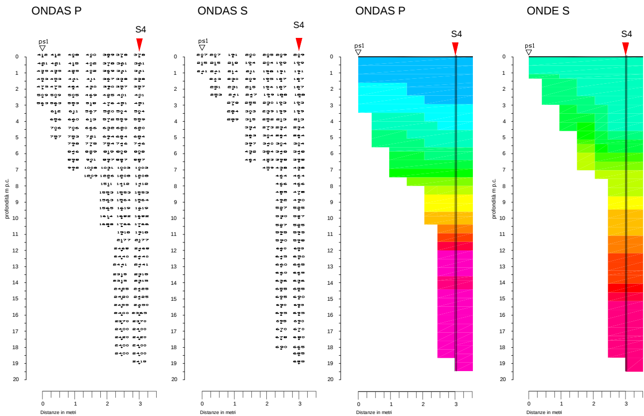
Pruebas sísmicas down-hole (cross-hole) en los sondeos geotécnicos para la detección de la velocidad de las ondas P y S
