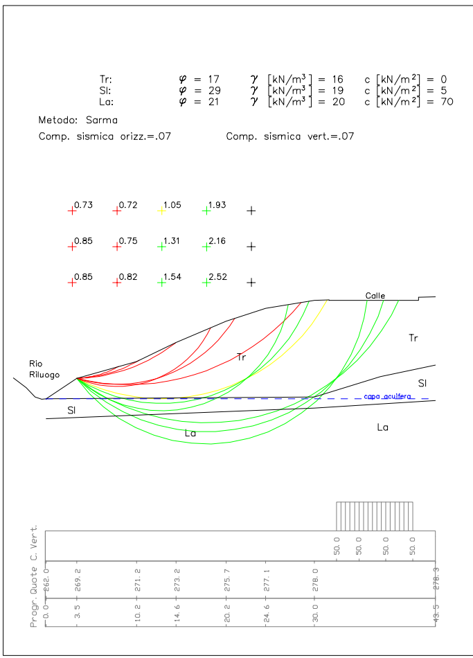
Verifica de la estabilidad de los vertientes enteresados para movimientos o inestabilidad
